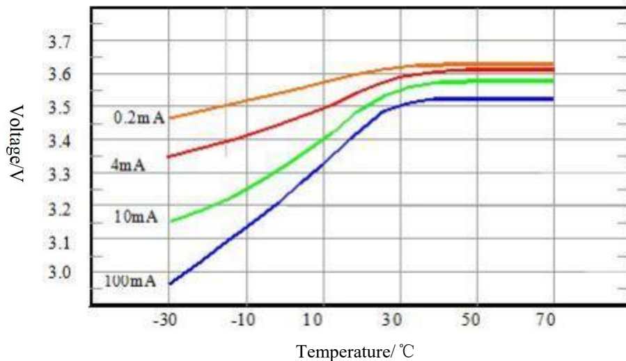
不同温度下电压平台特性图
