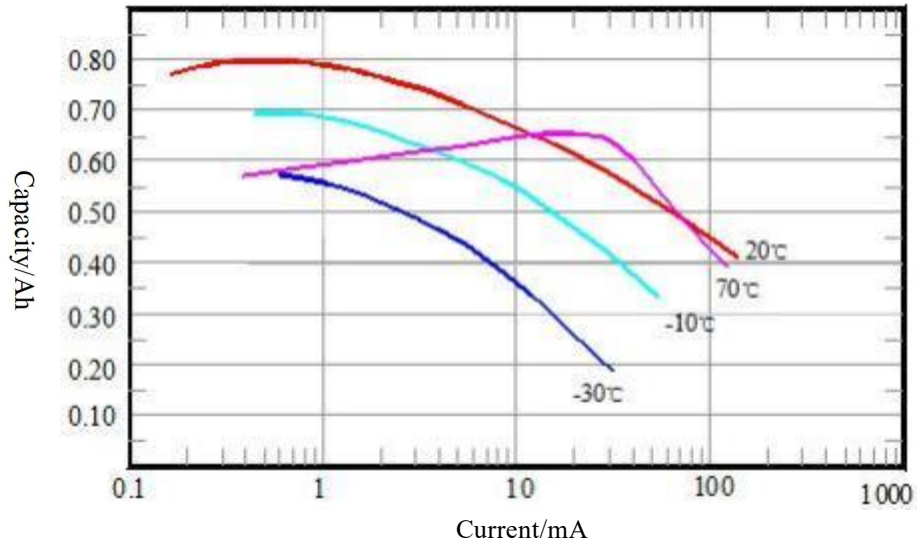
不同放电电流与放电容量特性图
