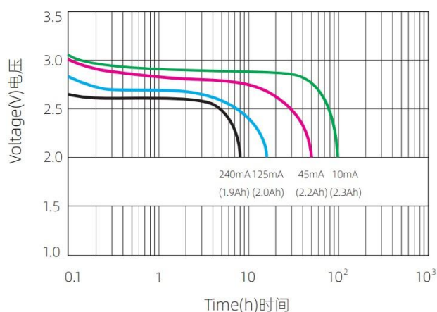
Discharge characteristic 放电特性 (25°C)
