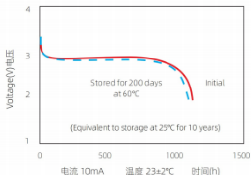
Storage characteristics 存储特性
