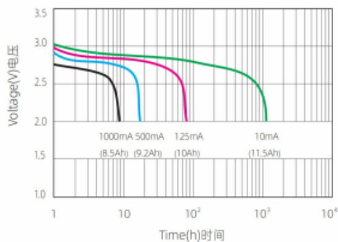
Discharge characteristic 放电特性 (25°C)
